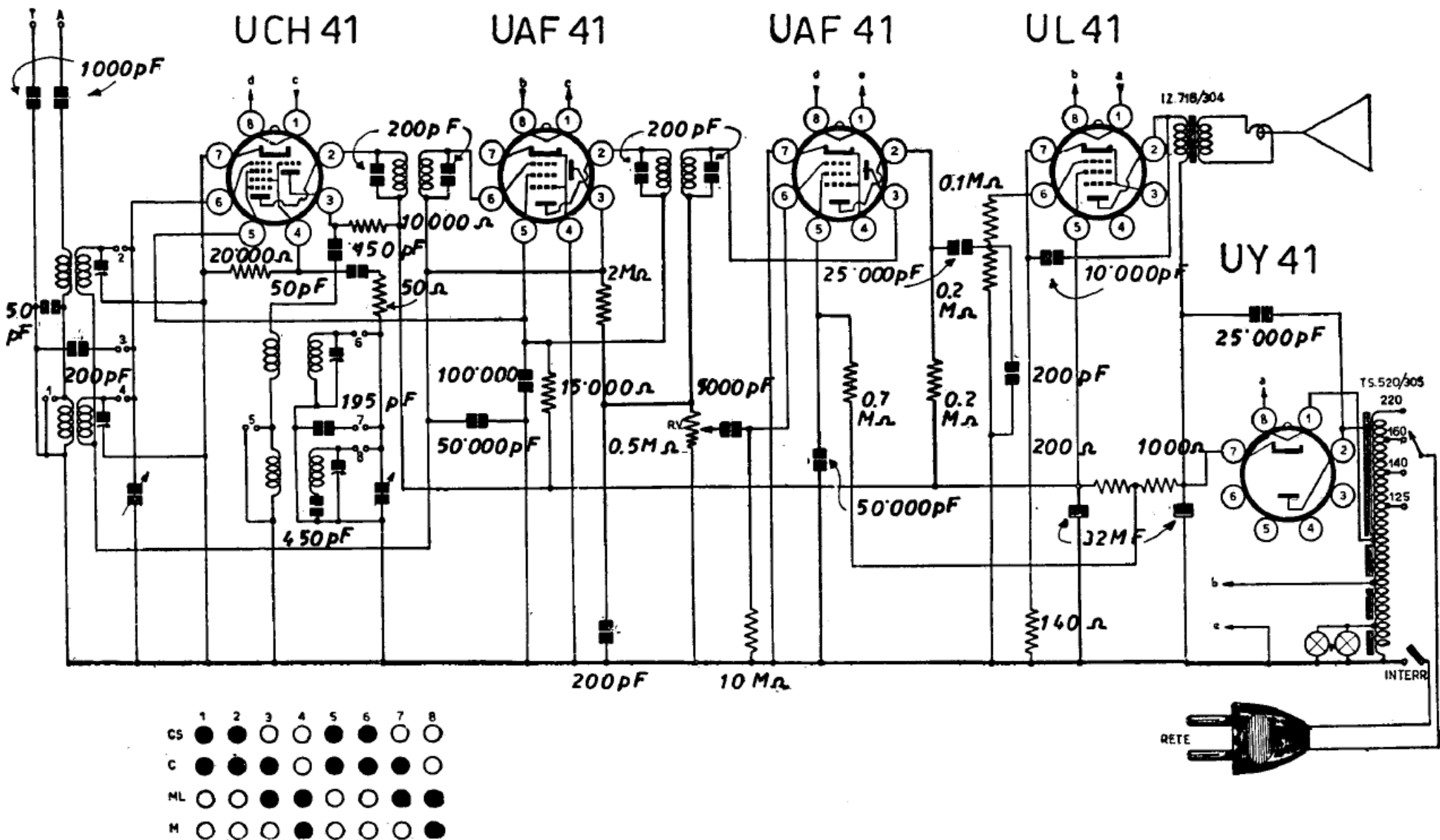
PHONOLA RADIO - Mod. 593 A e mod. 5507 - Valvola finale placca 174 V, schermo 154 V. Convertitrice placca pentodo 158, placca triodo 104 V, schermo 70 V. Valvola media frequenza, placca e schermo 70 V. MF a 470 kc. (Il mod. 5507 è a due gamme intere, medie e corte).
